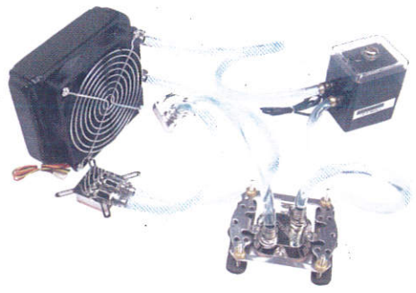
கி.பி.டி. லேர் கிலி கிளர் CPU Water Cooling System CPU நீர் குளிராக்கித் தொகுதி
